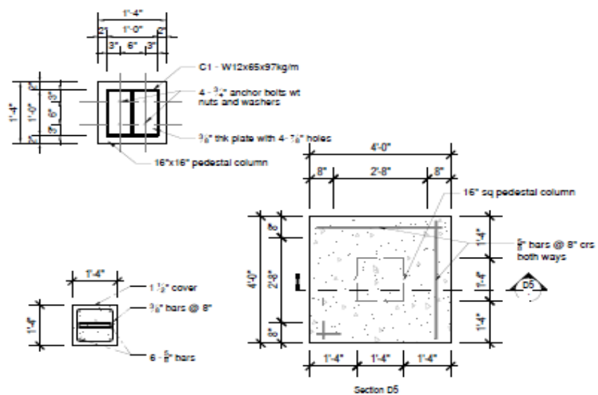
Section D5
