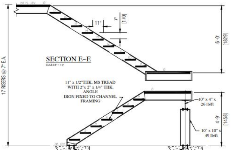
SECTION E~E SCALE: 3/8" = 1'-0" SECTION D~D SCALE: 3/8" = 1'-0"
