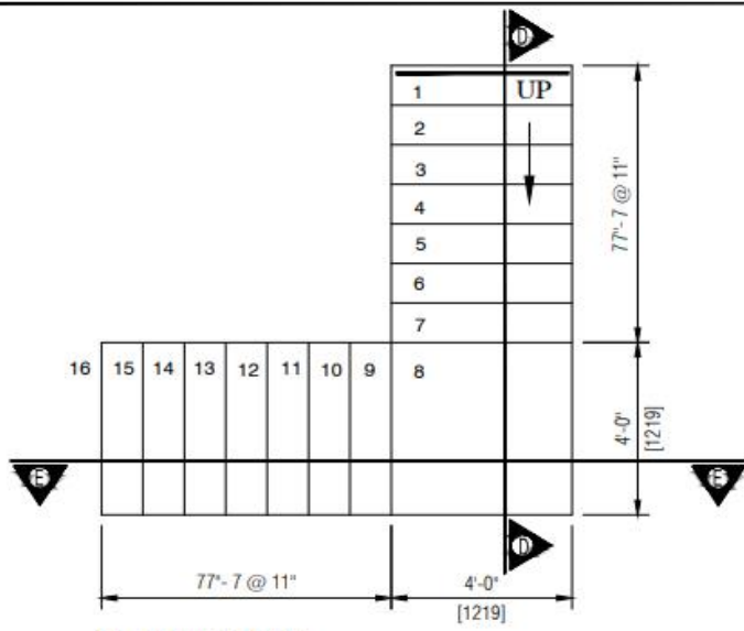
PLAN OF STAIR SCALE: 1/8" = 1'-0"
