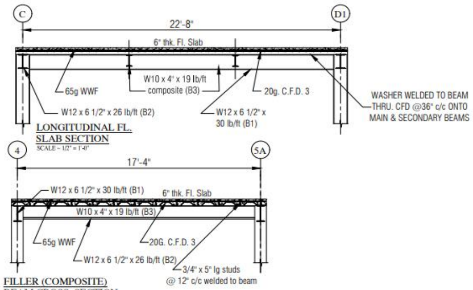
LONGITUDINAL FL. SLAB SECTION SCALE: 1/2" = 1'-0" FILLER (COMPOSITE) BEAM CROSS SECTION SCALE: 1/2" = 1'-0"
